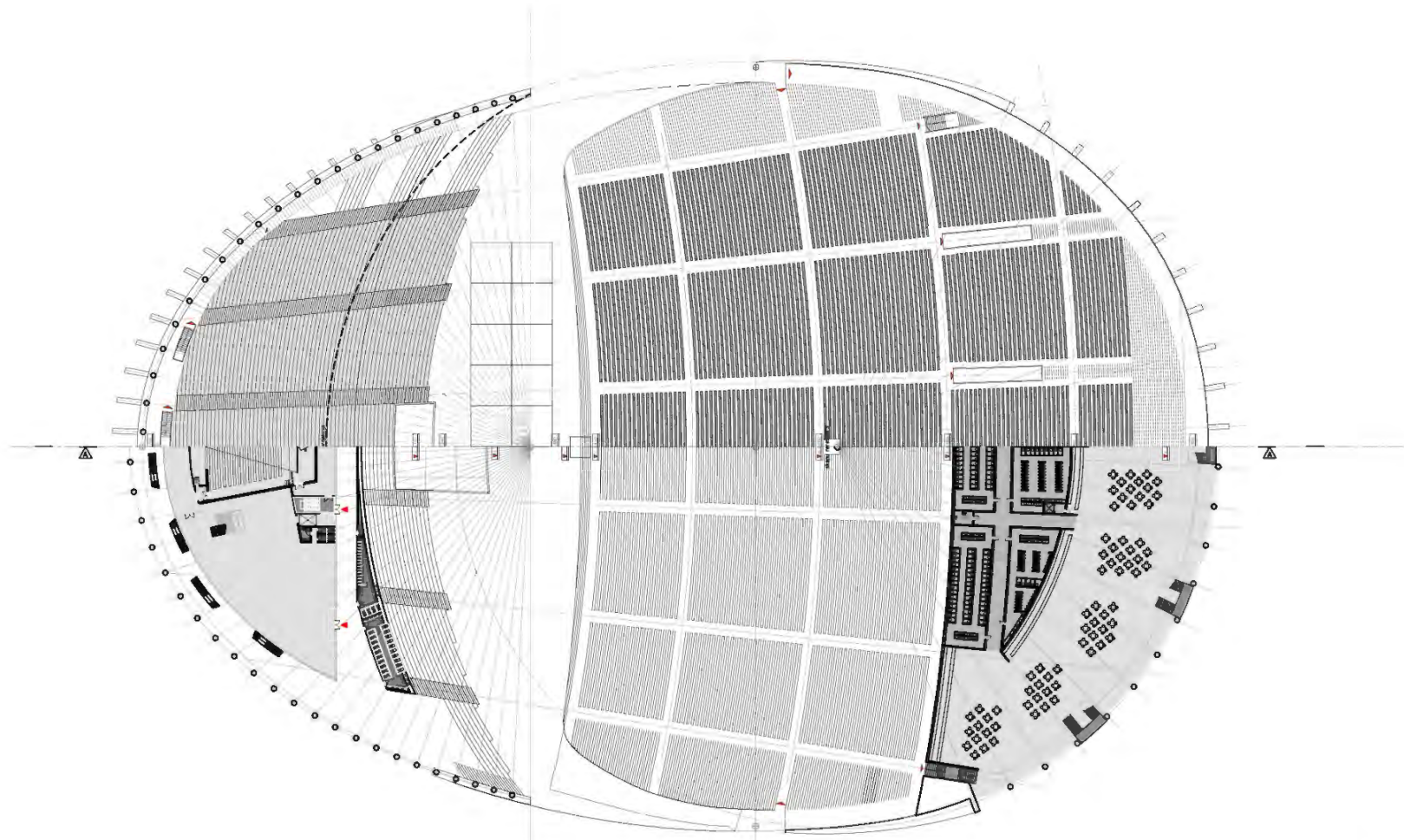
DZIESMU SVĒTKU ESTRĀDES PĀRBŪVE MEŽAPARKĀ Zemes un virsmas plāna shēma 2020
